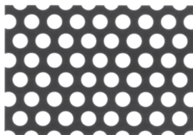
ø4,00 TD6,00 40%
